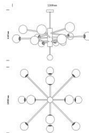
Dimensions fixation plafonnière
